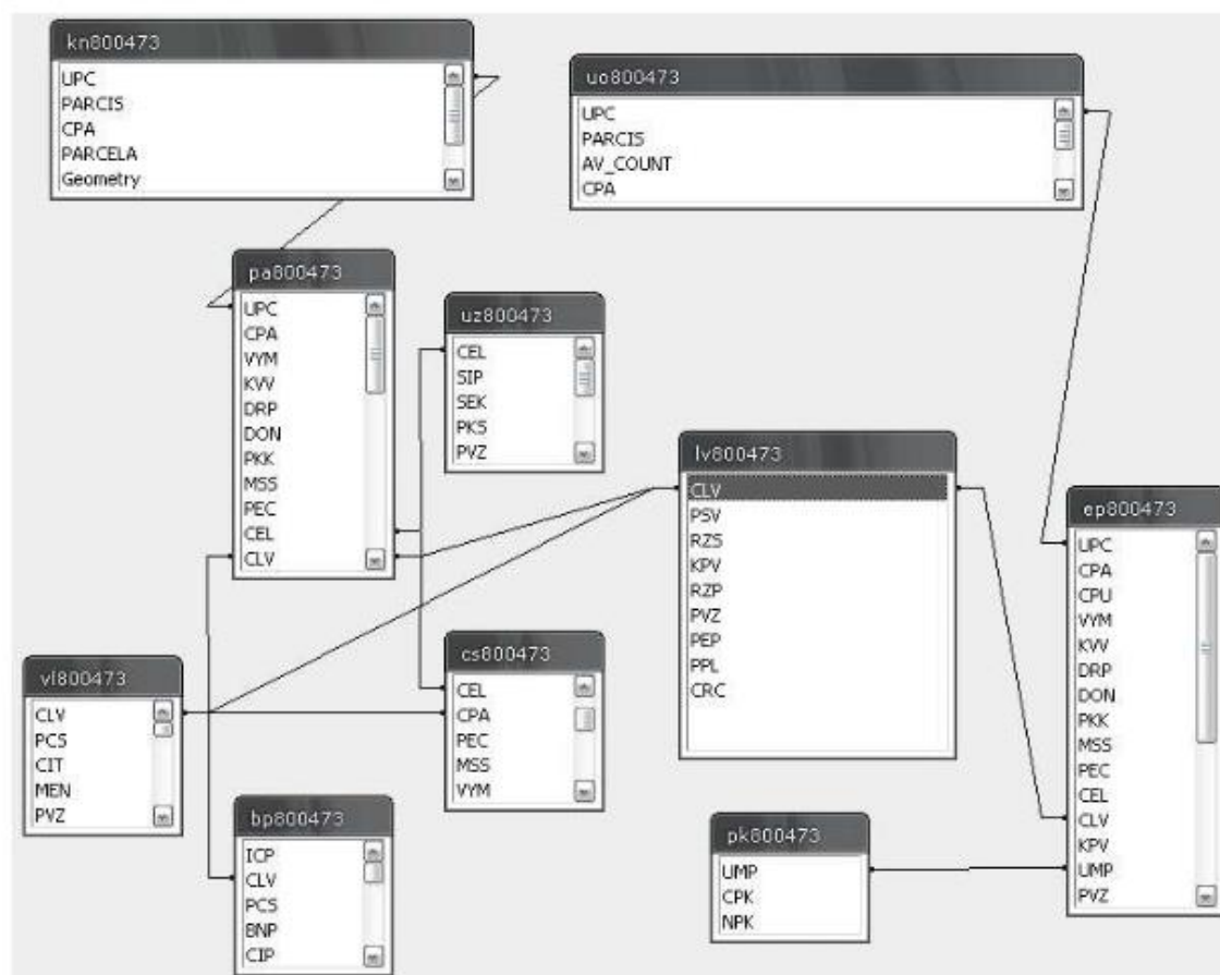
Obr. č.26: Relácie medzi tabuľkami a geometriou katastra nehnuteľností
