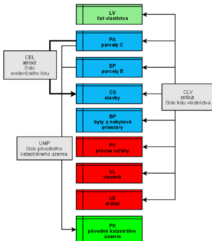
Obr. 7: Schéma údajového modelu SPIKN s väzbami
