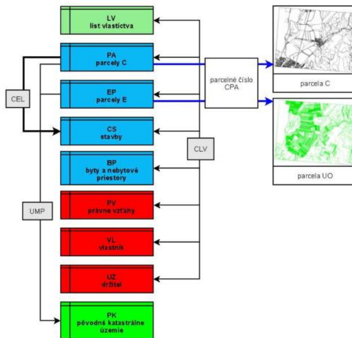
Obr. č.11:Schéma väzieb medzi SPIKN a SGIKN a v rámci nich.
